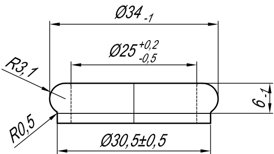
Венчик Масштаб 2:1
