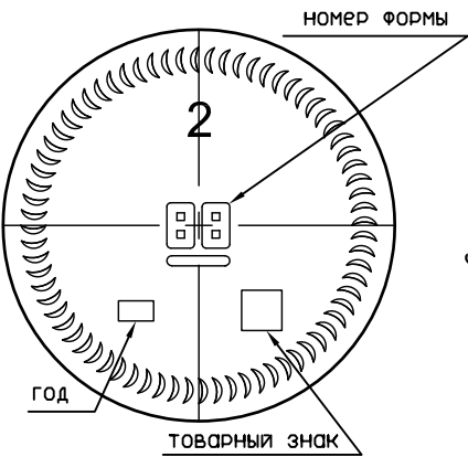
ВИД СНИЗУ
