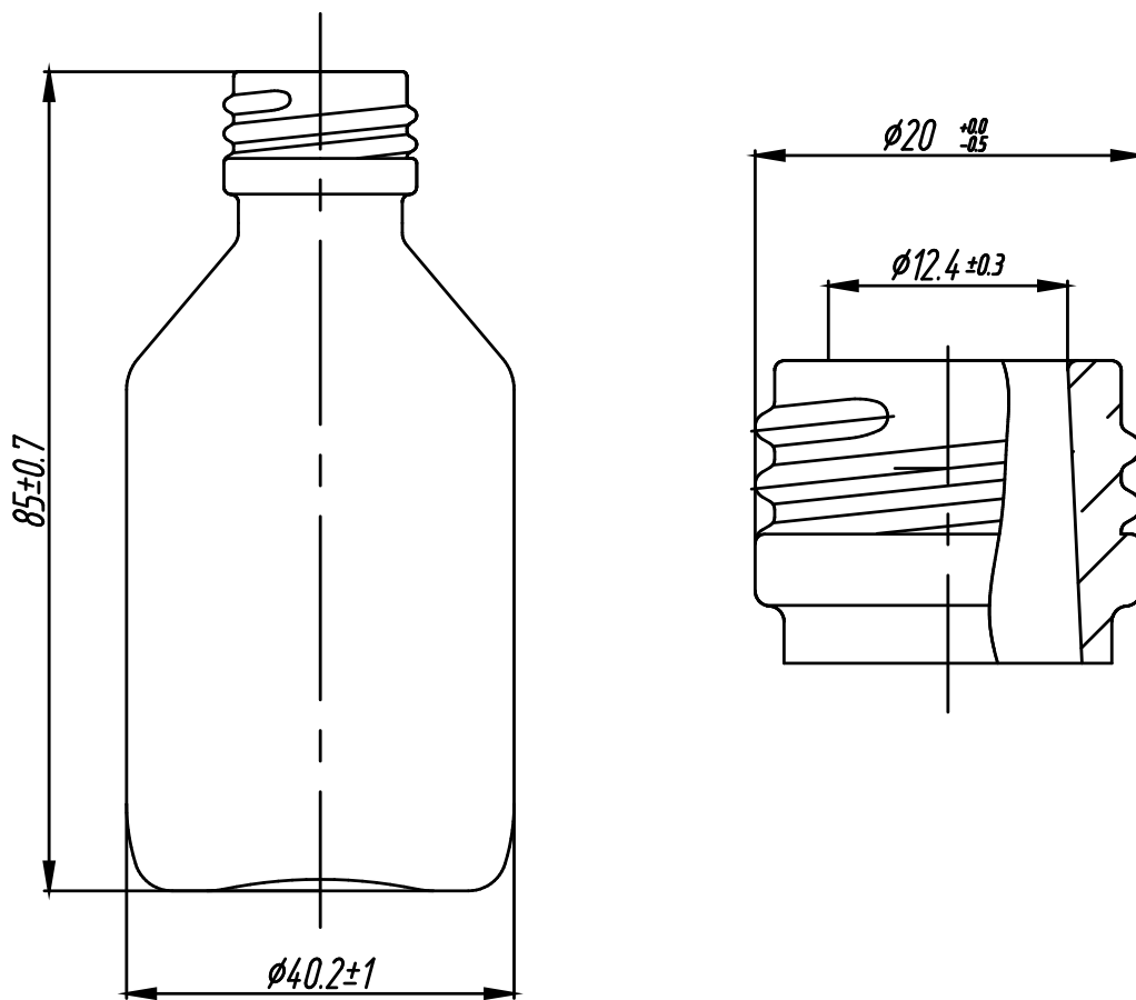
Венчик горловины типа ФВ-20
