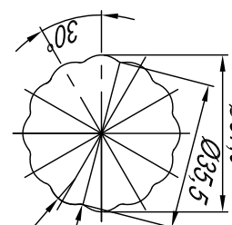
Б-Б Венчик ТОН-43 вид сверху (2:1)
